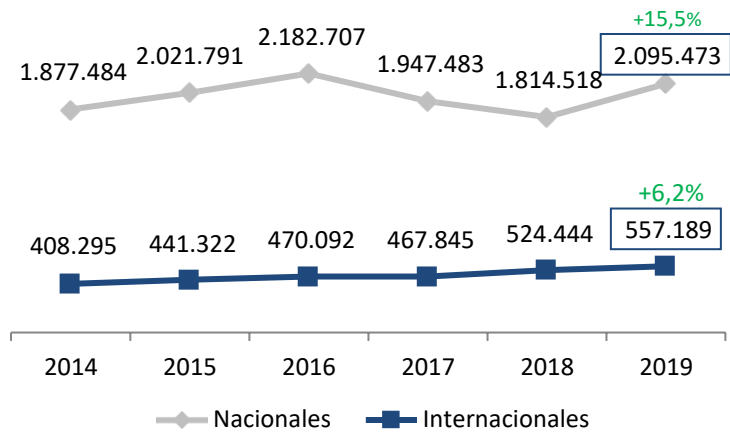
Gráfico 8. Número de Pasajeros movilizados en avión desde orígenes nacionales e internacionales con destino Cali (2014-2019)
