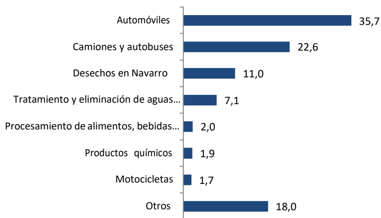
Gráfico 3. Principales emisores de GEI en Cali (%) (2015)
