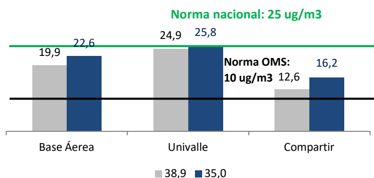
Gráfico 2. Niveles de PM 2,5 (µg/m 3 ) en Cali (2018 - 2019)
