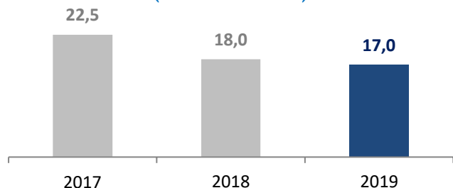
Gráfico 13. Número de horas por usuario en que se suspendió el servicio de energía eléctrica en Cali (2017 - 2019)
