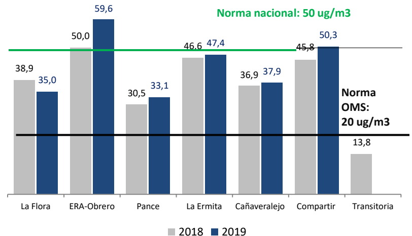
Gráfico 1. Niveles de PM10 ( \mu\text{g}/\text{m}^3 ) en Cali (2018 – 2019)*
